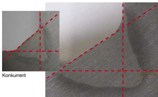
Elgacore® Matrix svetsinträngning
