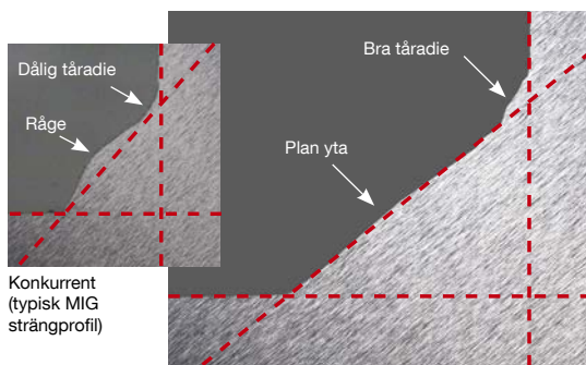
Elgacore® Matrix svetsinträngning (fogprofil)
